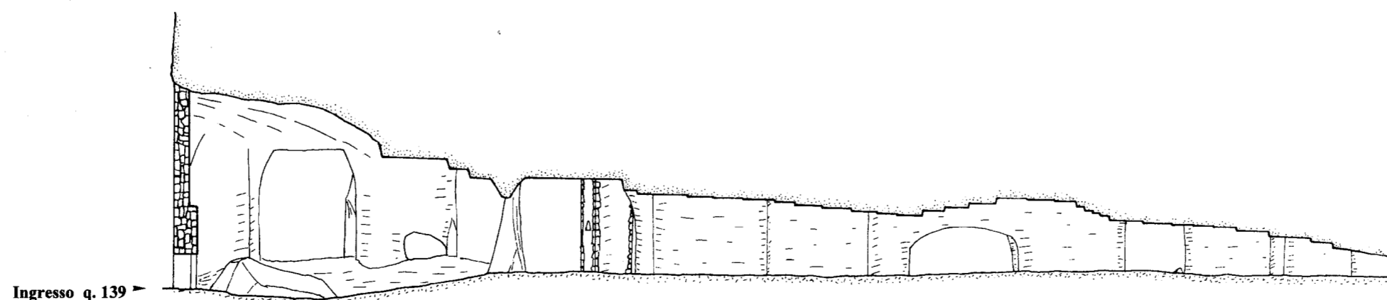
SEZIONE LONGITUDINALE
